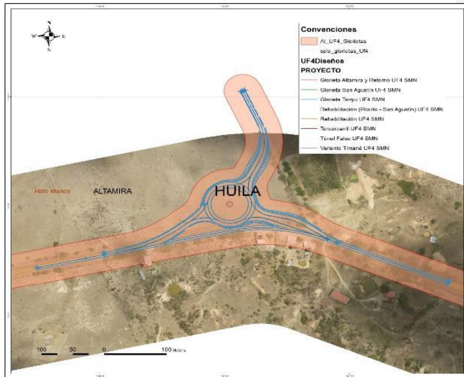
Figura 5. 5. Intersección Tarqui UF4 K41+380-42+018
