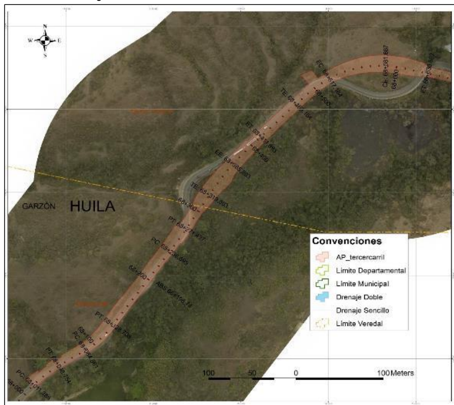
Figura 5. 9. Área afectación tercer carril UF4 K68+000 – K 68+630
