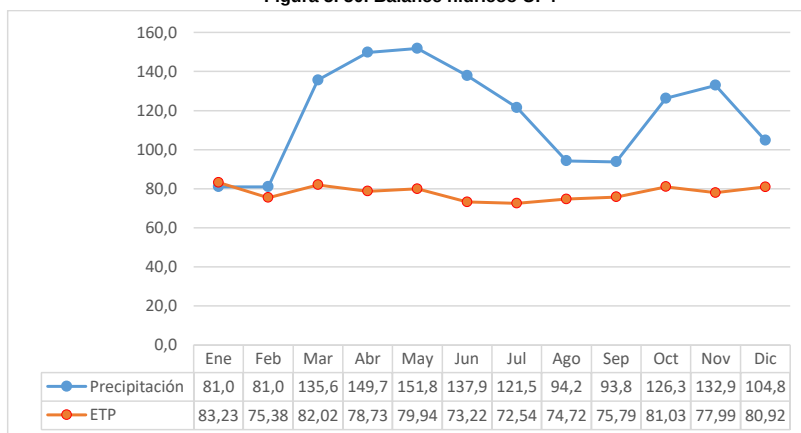
Figura 5. 50. Balance hidrico UF4
