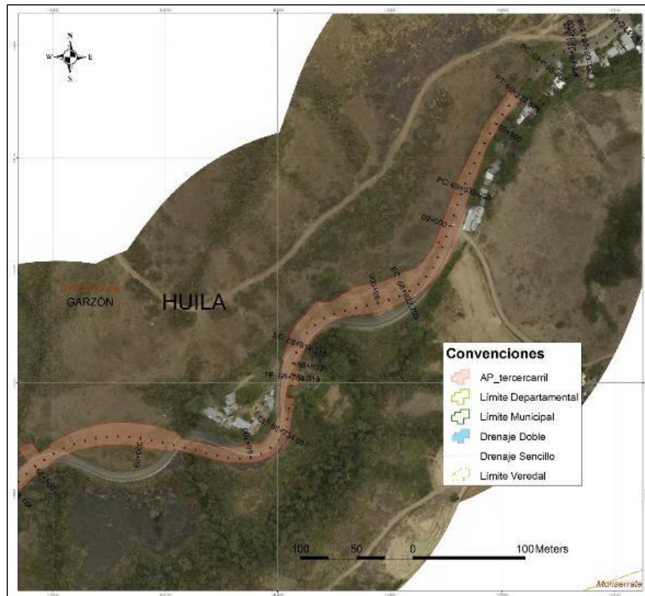
Figura 5. 10. Área afectación tercer carril UF4 K68+500 – K 69+130
