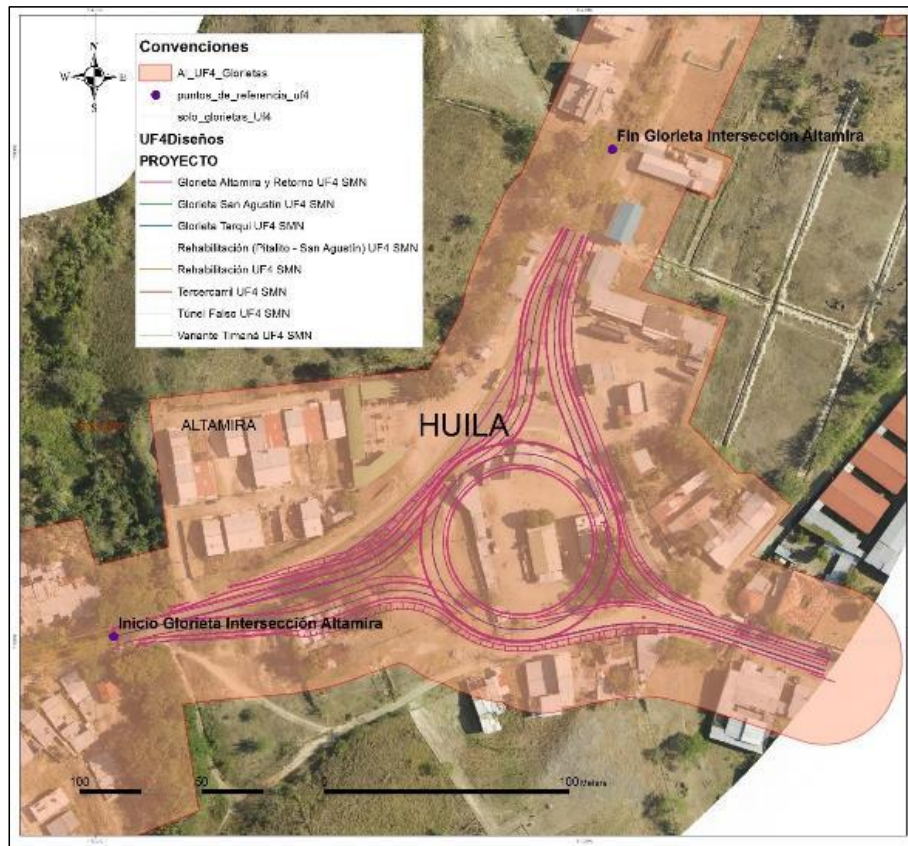
Figura 5. 6. Intersección Altamira K44+616 - K44+918 UF4
