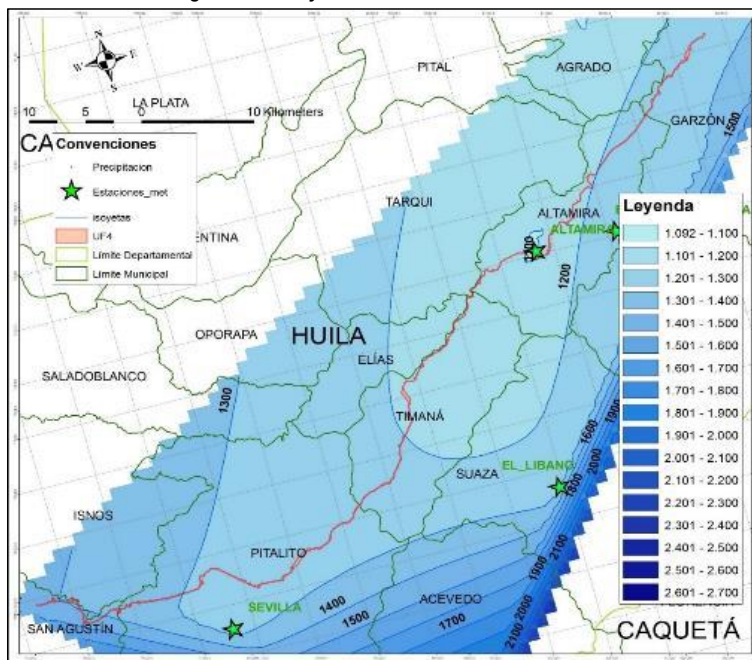
Figura 5. 45. Isoyetas en el área de influencia UF4
