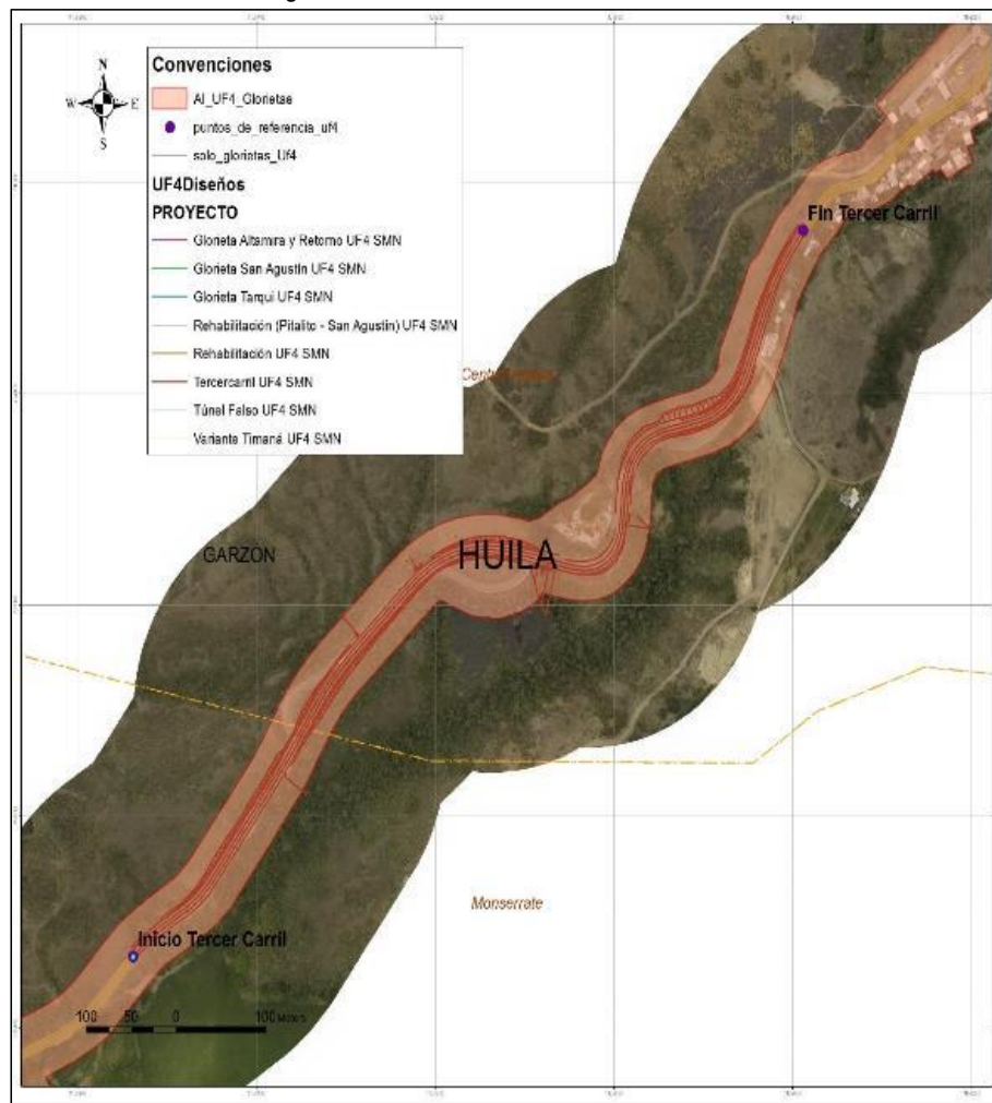
Figura 5. 8. Tercer Carril UF4 K 68+012 – K69+130
