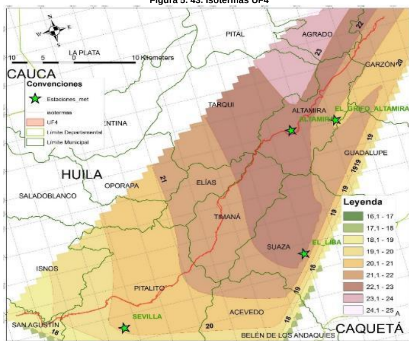
Figura 5. 43. Isotermas UF4
