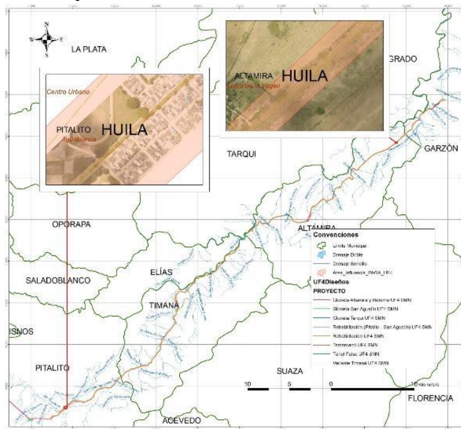
Figura 5. 3. UF4 Sector rehabilitación Pitalito hasta Garzón 0+000 – K70+000
